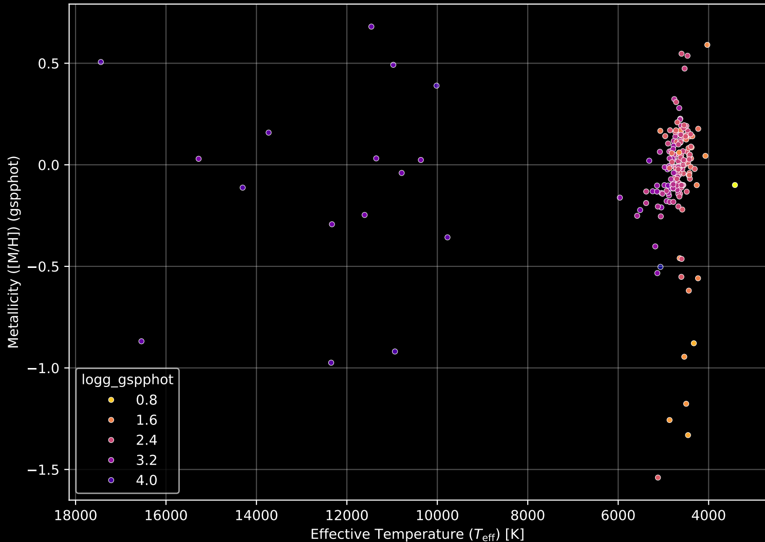
APOGEE DR17 Field: [045-06] Stellar Population Parameters (n= 187)
